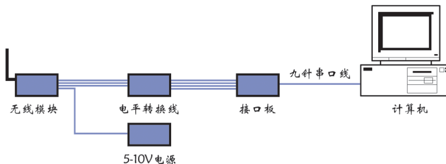
模块设置及测试连接示意图
