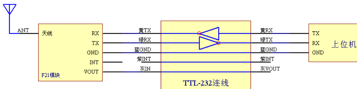
上位机为RS232电平时的连接
