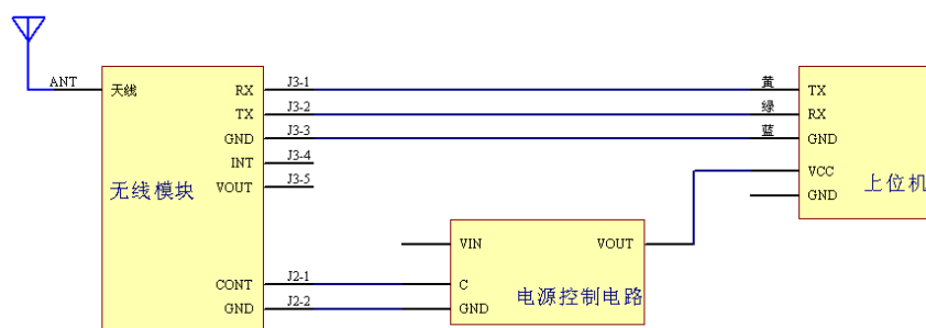
省电方式下空间唤醒控制电源电路的连接方法
