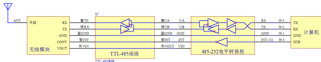
使用 485 电平转换线时的连接
