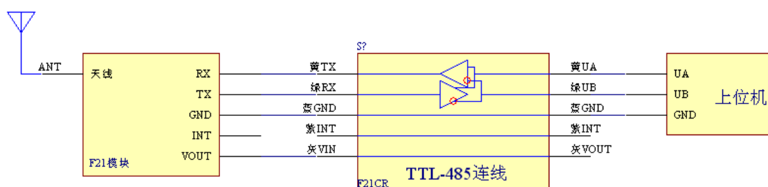
上位机为RS485电平时的连接
