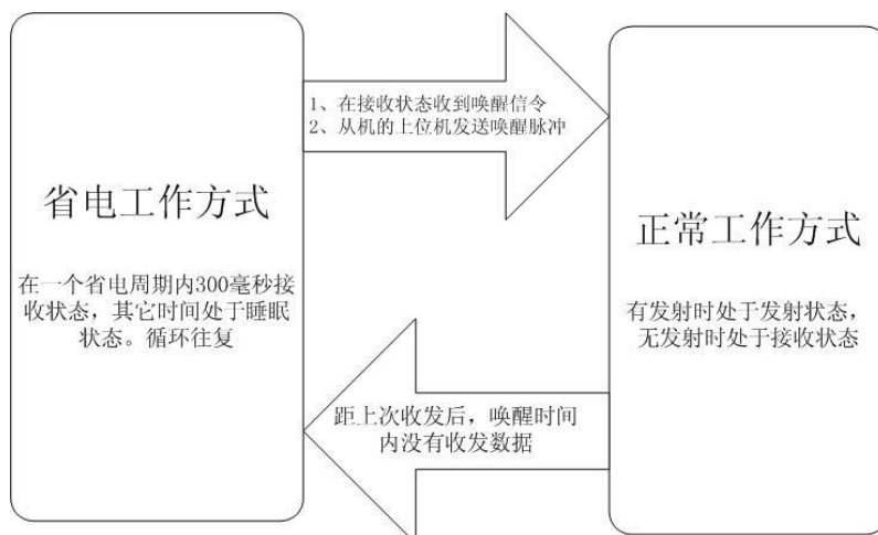
省电模式下两种工作方式的转换
