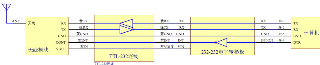
使用 232 电平转换线时的连接
